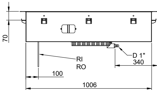
Zij aanzicht
